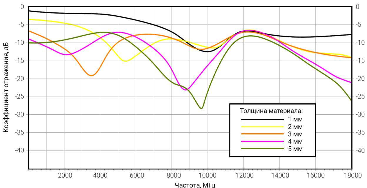
Рисунок 1 – Радиопоглощающие свойства герметика ЗИПСИЛ 410 РПМ-Л для толщин слоя от 1 до 5 мм. График коэффициента отражения плоской волны
