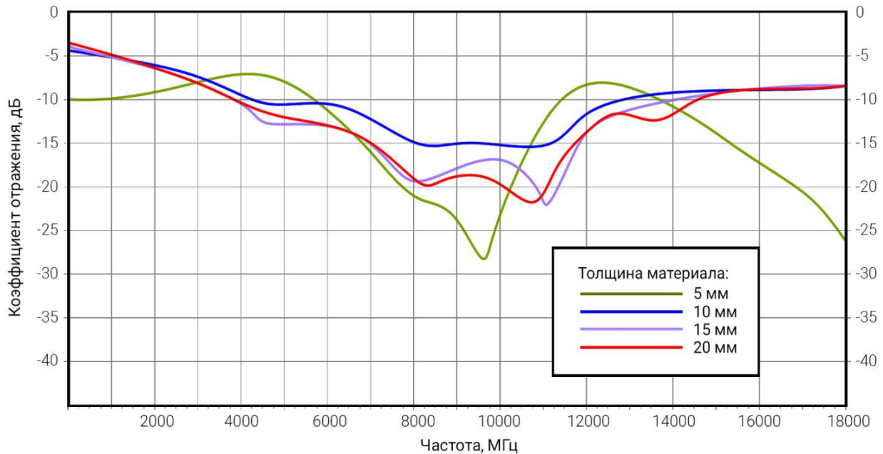
Рисунок 2 – Радиопоглощающие свойства листового материала ЗИПСИЛ 601 РПМ-01 для толщин от 5 до 20 мм. График коэффициента отражения плоской волны
