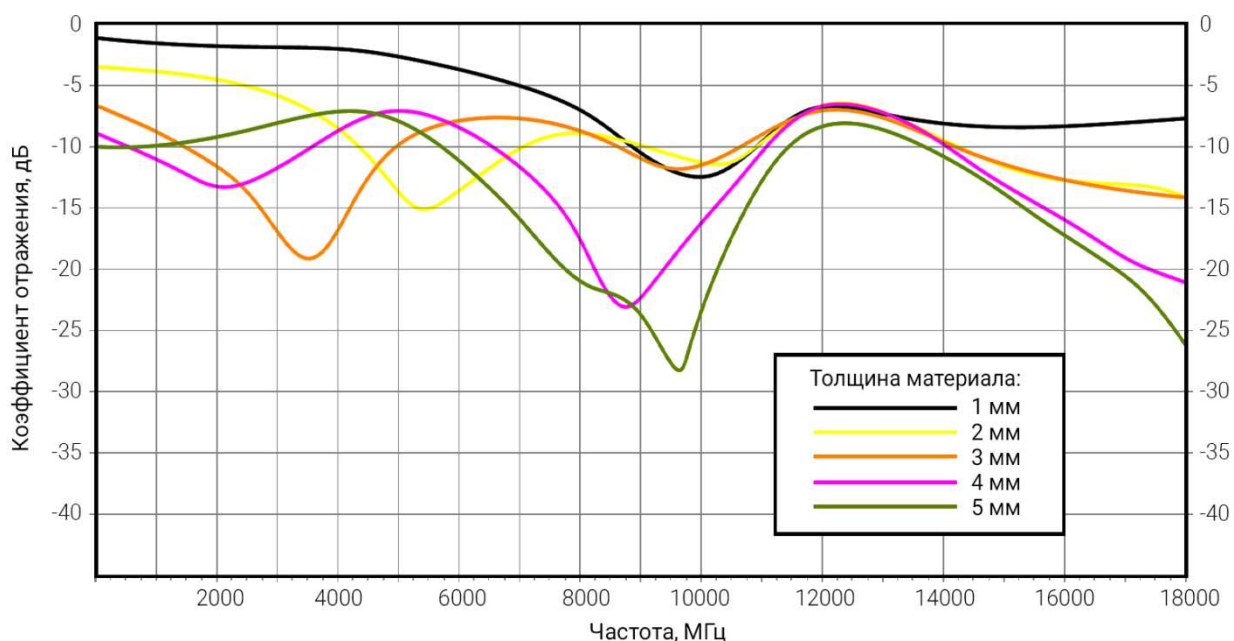
Рисунок 1 – Радиопоглощающие свойства листового материала ЗИПСИЛ 601 РПМ-01 для толщин от 1 до 5 мм. График коэффициента отражения плоской волны
